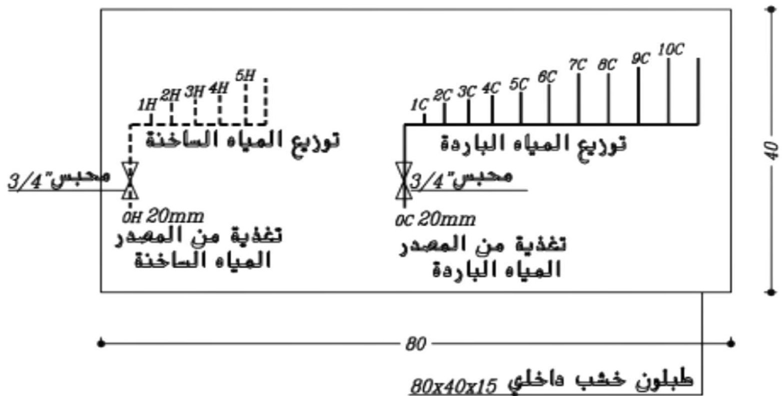
مقطع تفصيلي للطبلون الرئيسي للمياه الباردة و الساخنة
